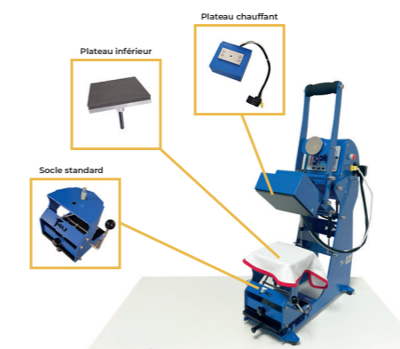
TMax CPA15 Presse à patch
