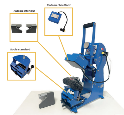
TMax CCH15 Presse à chaussure
