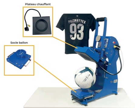
TMax CBA13 Presse à ballon
